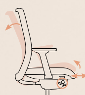
Synchrone Pro + : réglage manuel de la tension du dossier via une manette sur le côté facilitant l'usage, avec ajout de la translation d'assise
